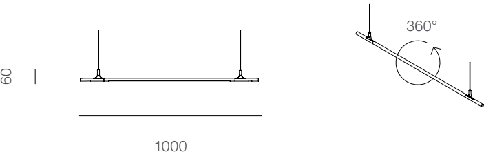
PENDANT 2 SECTIONS
